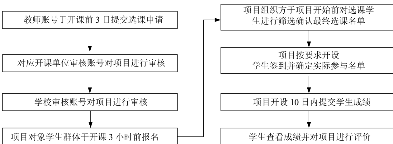
图 1 第二、三课堂信息管理系统管理流程
